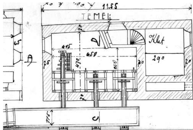
Dovjakov mlin, načrt iz leta 1924, tloris. Načrt je delo Matevža Demšarja iz Poljan 53 (ZAL Škofja Loka, ŠKL 13, a. e. 1, Vodnopravni spisi).
