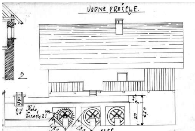
Dovjakov mlin, načrt iz leta 1924, pogled z vodne strani. Načrt je delo Matevža Demšarja iz Poljan 53 (ZAL Škofja Loka, ŠKL 13, a. e. 1, Vodnopravni spisi).
