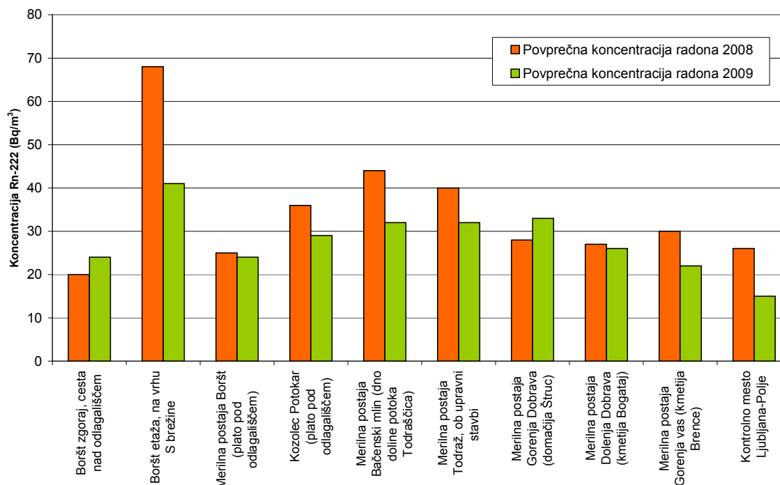
Diagram 3: Povprečne letne koncentracije Rn-222 v vzdolžnem profilu Merilna postaja Boršt Bačenski mlin – Gorenja vas, detektorji sledi, leti 2008 in 2009
