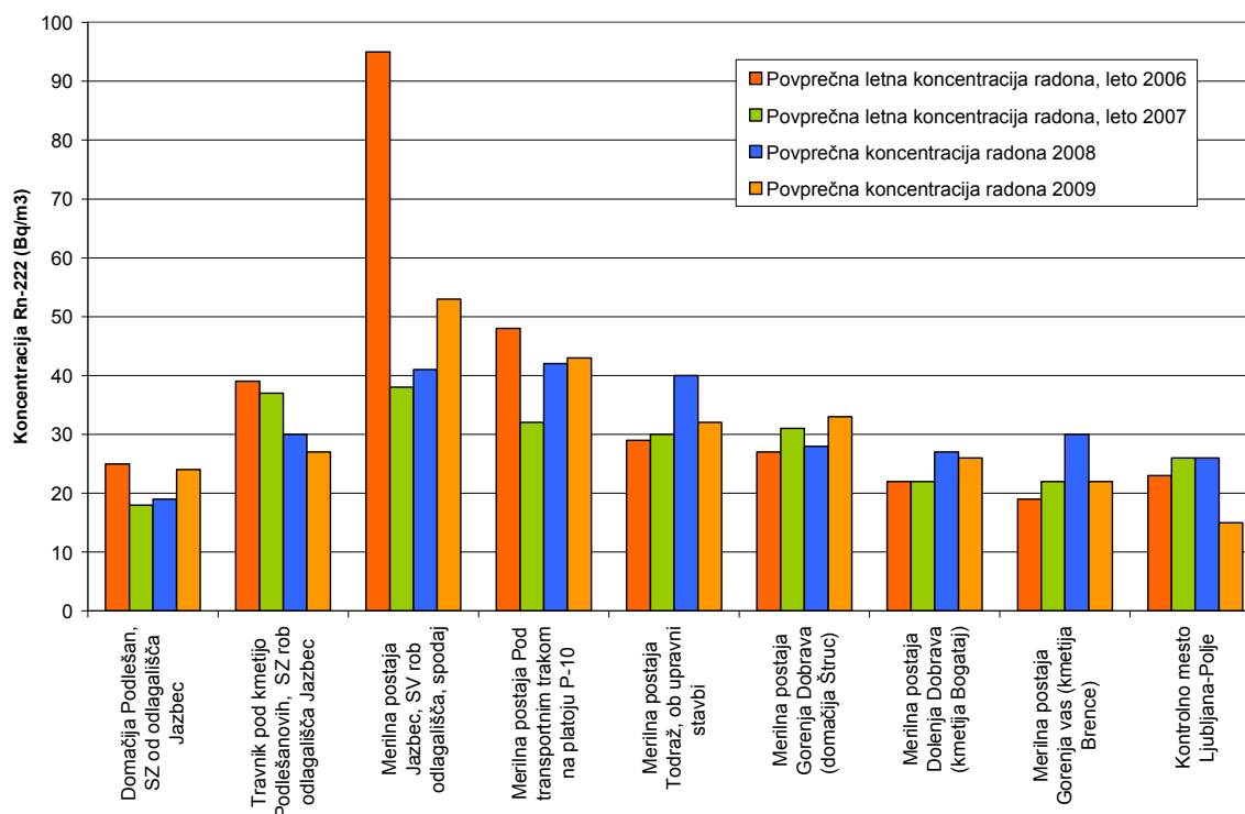
Diagram 2: Povprečne letne koncentracije Rn-222 v vzdolžnem profilu stanovanjska hiša Podlešan – odlagališče Jazbec – Gorenja vas, detektorji sledi, leta 2006-2009
