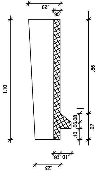
VZDOLŽNI REZ
