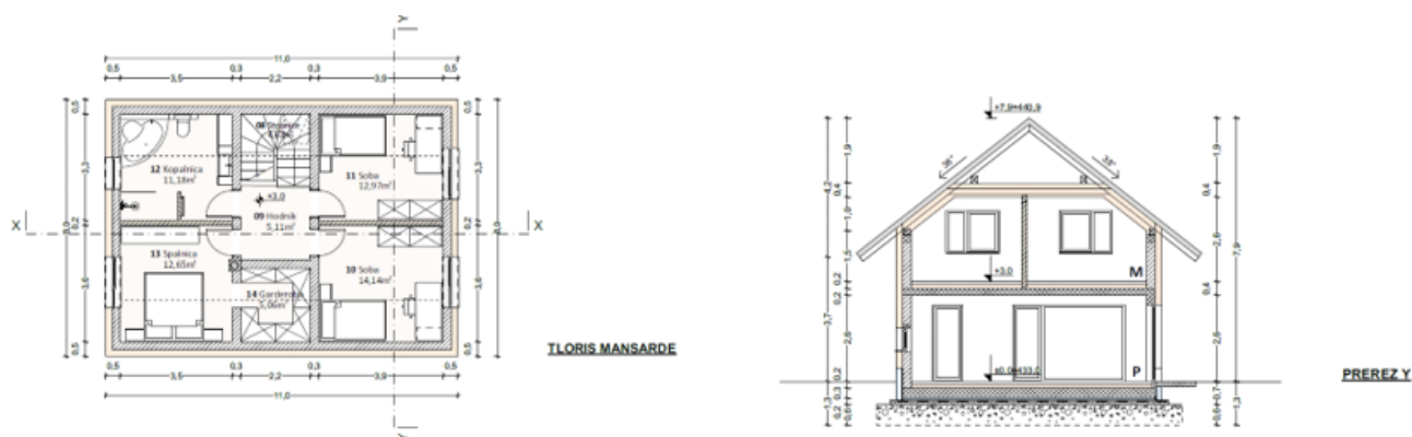
Slika 16: Tloris in prerez stanovanjske stavbe (izsek iz DGD)
