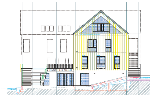
Načrt južne fasade novega kulturnega doma (arhiv ArheoAlpe, zavod za kulturo, izobraževanje in turizem Bohinj)
