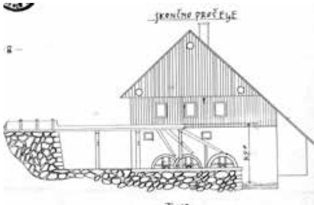
Bukov Vrh 8: Drnovškov mlin, posnetek stanja decembra 1923. Avtor risbe in vir kot pri sliki za Hotovljo 1.
