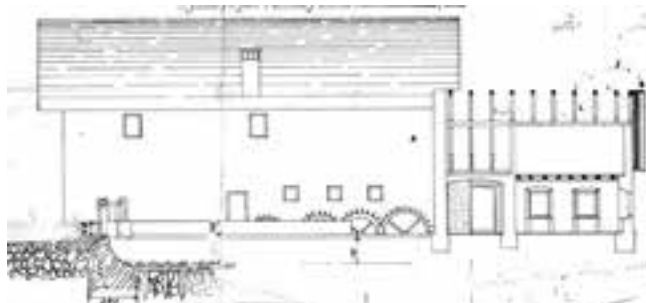
Hotovlja 3: Vosoški mlin, pogled z vodne strani, voda priteka z leve. Drugo kot pri sliki za Hotovljo 1.
