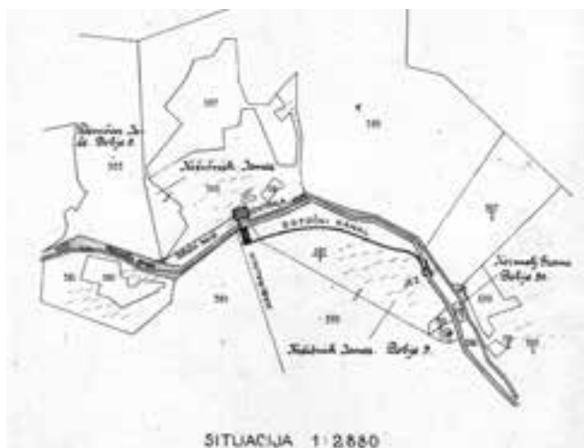
Elektrarna, umestitev v prostor, narisano v biroju dr. Miroslava Kasala leta 1919. Vir kot pri sliki za Hotovljjo 1.
