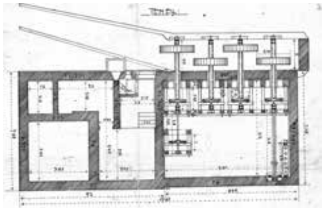
Bukov Vrh 9: Kisovski mlin, tloris, posnetek stanja julija 1922. Voda je pritekala z desne. Avtor risbe in vir kot pri sliki za Hotovljo 1.
