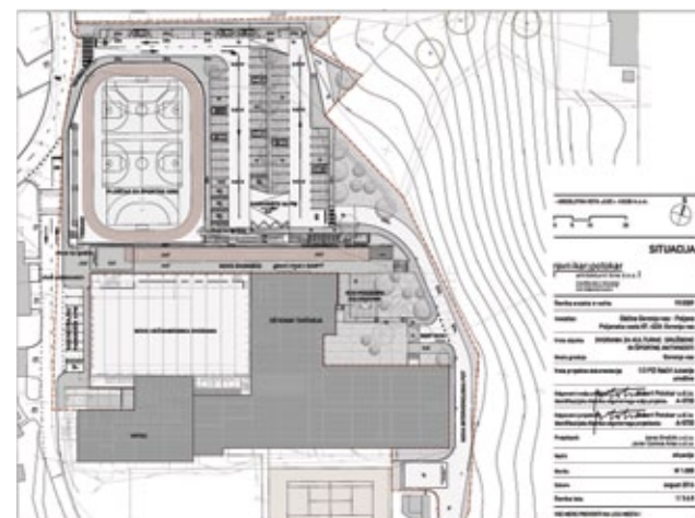
Situacija športne dvorane
