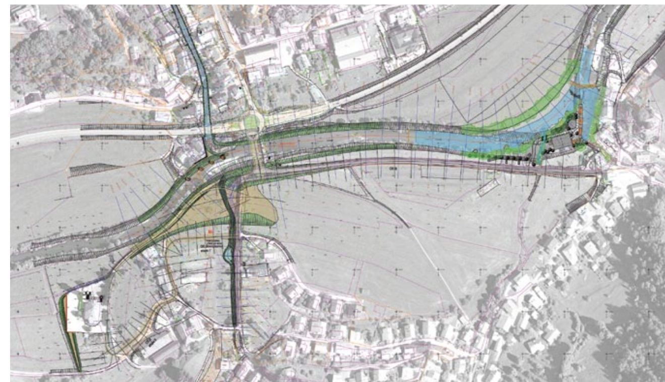
Zasnova protipoplavnih ureditev v Poljanah
