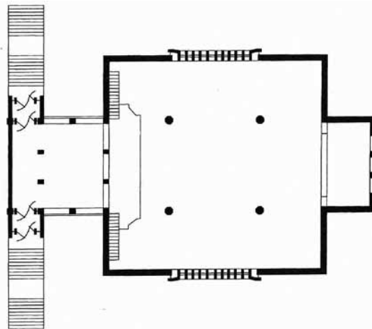
Prvotni Bitenčev tloris nove cerkve v Predmostu (vir neznan)
