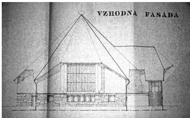
Vzhodna fasada cerkve – prvi načrt brez zvonika (vir: SI_ZAL_ŠKL/0141 fond SO Škofja Loka, številka tehnične enote 40)
