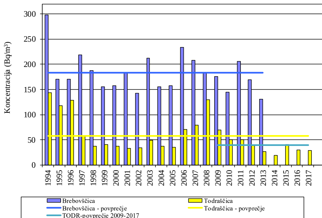
Slika 7: Povprečne letne koncentracije U-238 v Brebovščici in Todraščici PO
