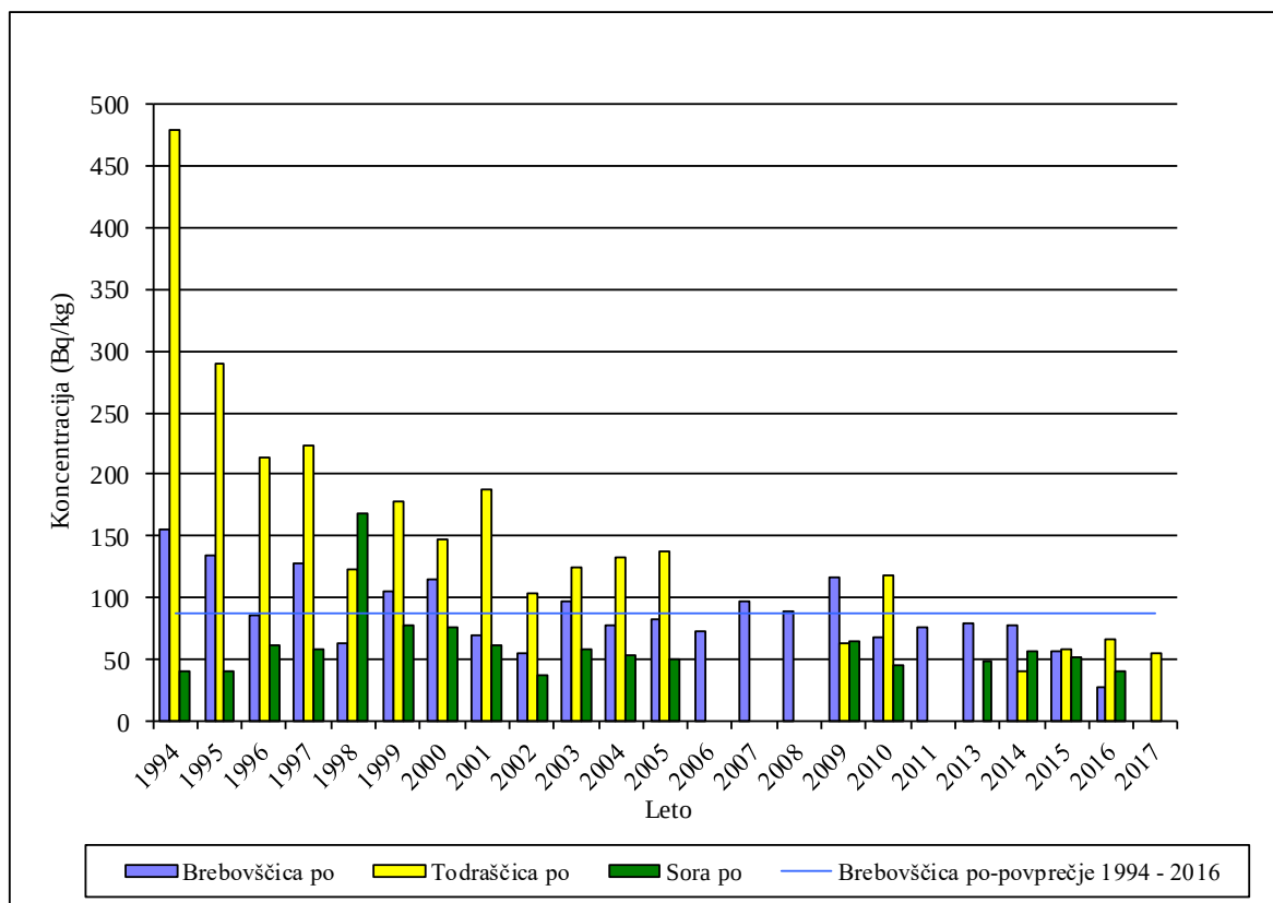
Slika 15: Koncentracija Pb-210 v sedimentih voda v okolici RŽV
