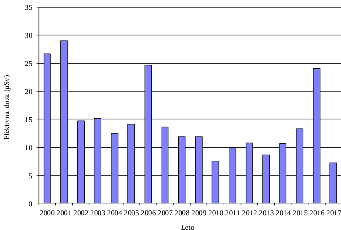
Slika 20: Letne efektivne doze zaradi pitja vode (Brebovščica) za odraslega prebivalca iz okolice RŽV
