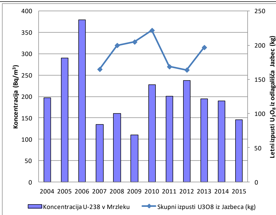
Slika 12: Koncentracije U-238 v izviru Mrzlek (Bq/m 3 ) in letni izpusti U 3 O 8 (kg) iz odlagališča Jazbec
