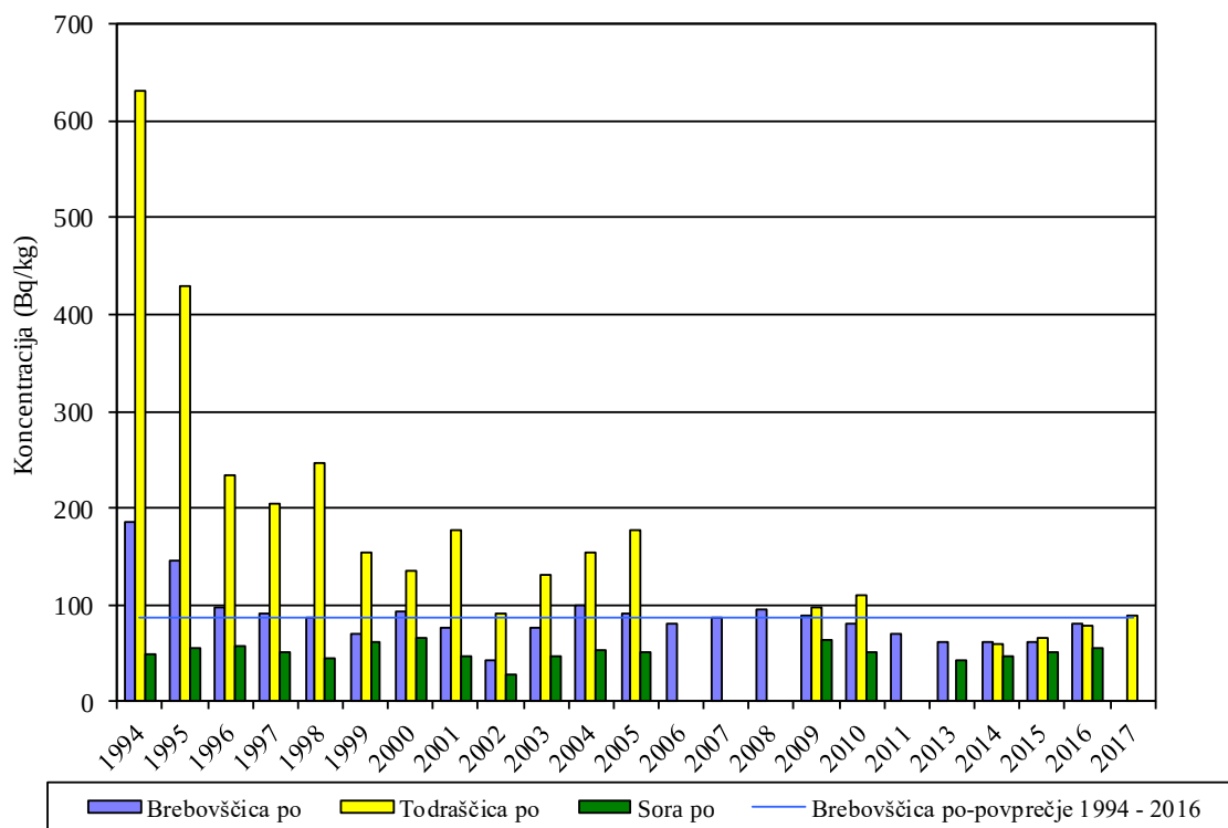
Slika 14: Koncentracija Ra-226 v sedimentih voda v okolici RŽV
