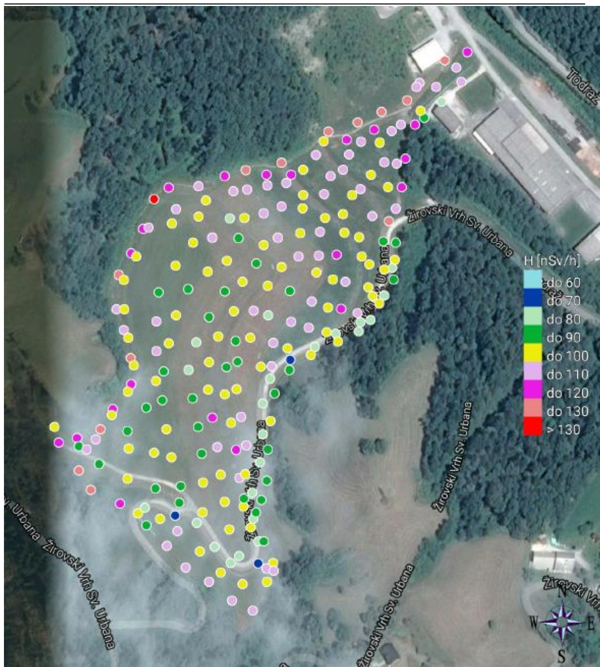
Slika 17: Meritve hitrosti doze zunanjega sevanja gama na površini odlagališča Jazbec. Meritve na višini 1 m, povprečevalno območje 25 m. Meritve je izvedel M. Eržen iz Agencije za radioaktivne odpadke, poročilo Meritve doznega polja na odlagališču Jazbec, oznaka ARAO-09-01-003/ME/17-SVS-06, maj 2017..
