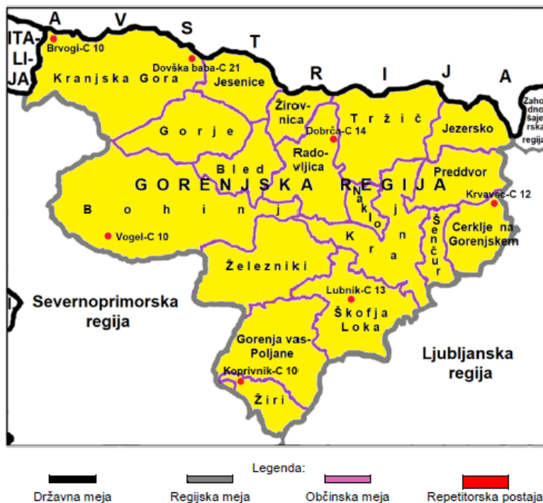
Slika 8: Repetitorske postaje s kanali sistema ZA-RE
